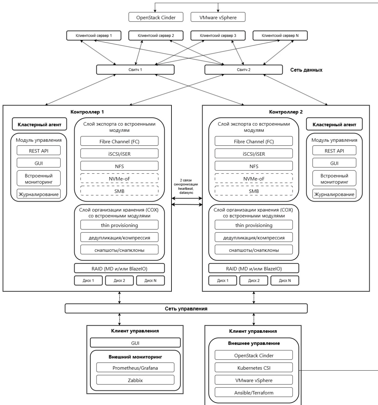
Рисунок 1 - схема архитектуры управляющего ПО BlazeX
