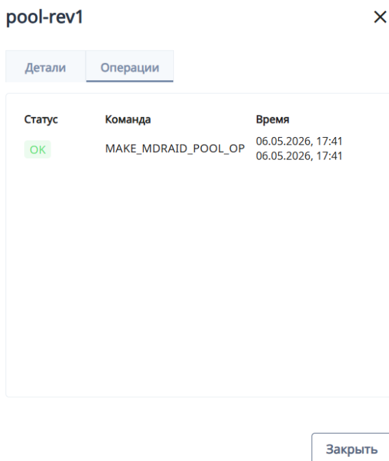
Рисунок 2.25 – Вкладка «Операции»
