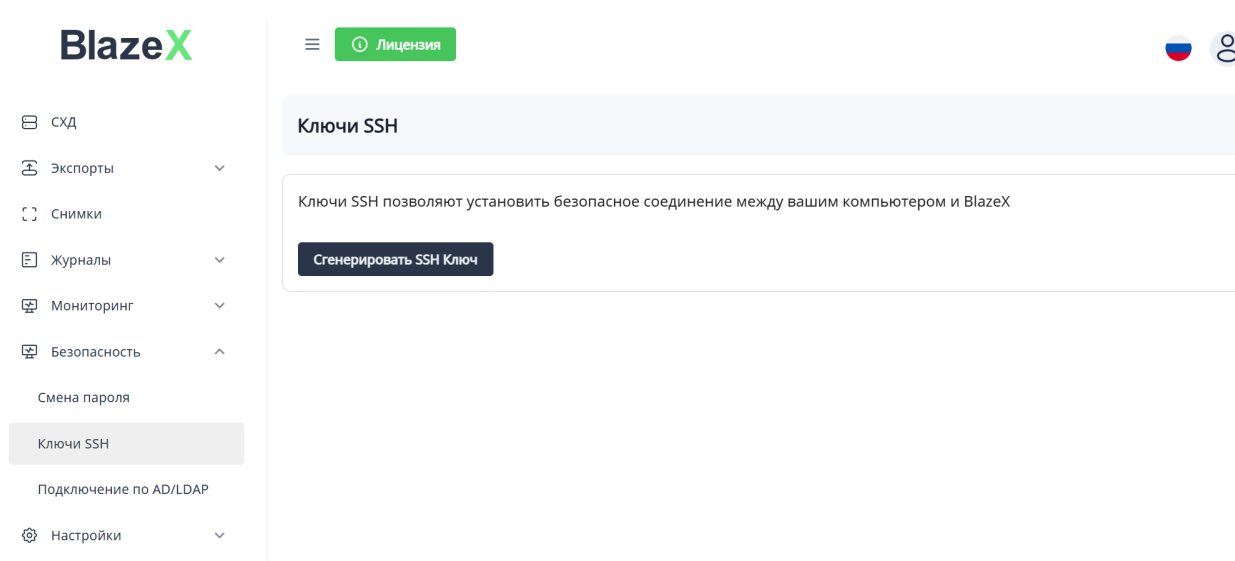
Рисунок 1.13 – Раздел «SSH-ключи»
