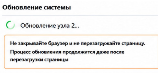
Рисунок 1.31 – Обновление узла 2
