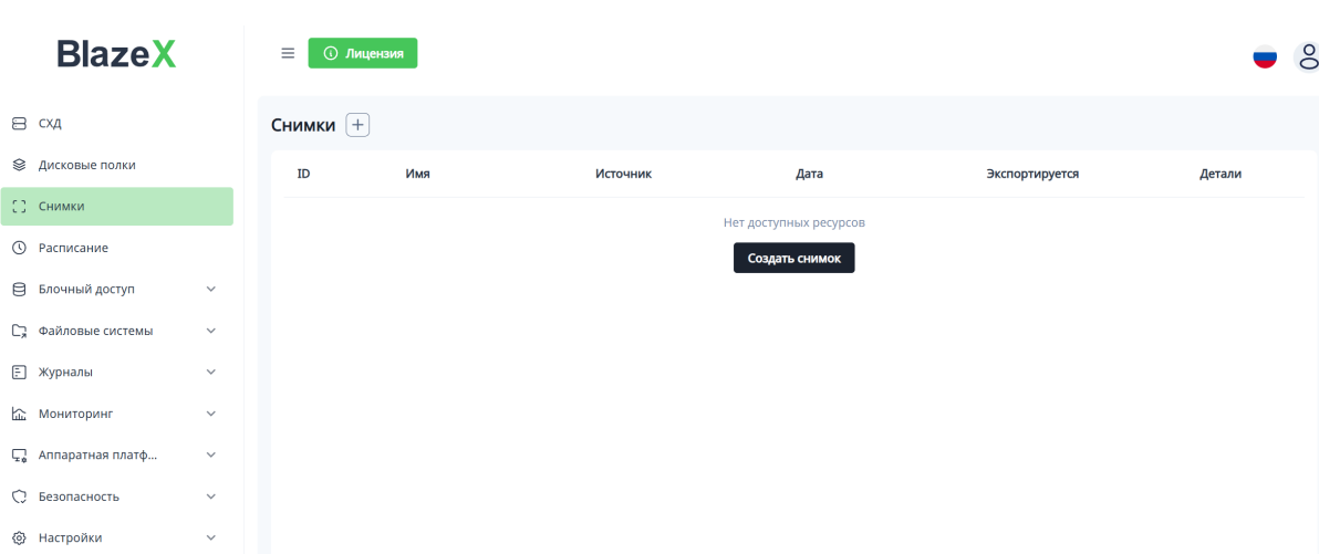
Рисунок 4.1 – Окно «Снимки»
