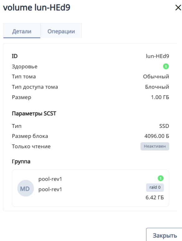
Рисунок 2.45 – Вкладка «Детали»
