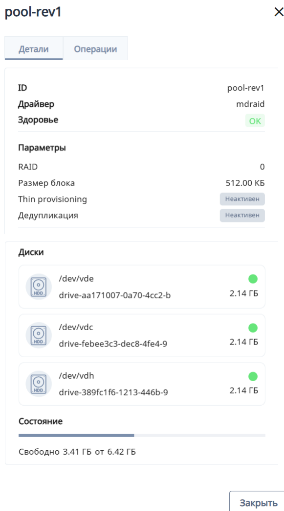
Рисунок 2.24 – Вкладка «Детали»
