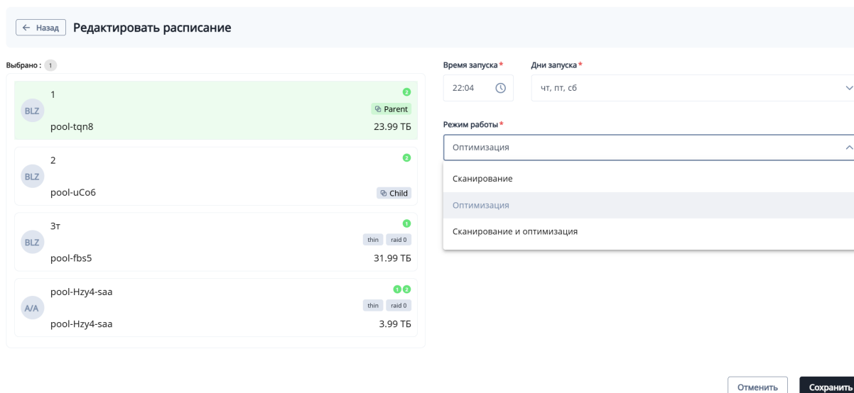
Рисунок 5.9 – Редактирование расписания
