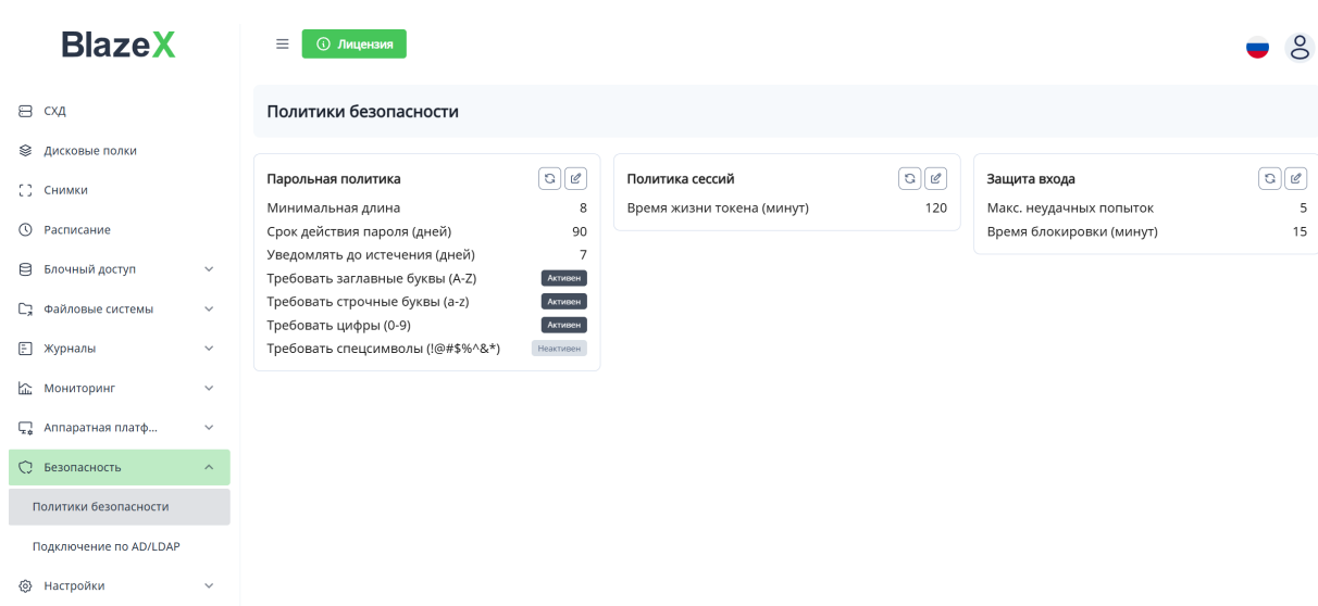
Рисунок 11.1 – Политики безопасности
