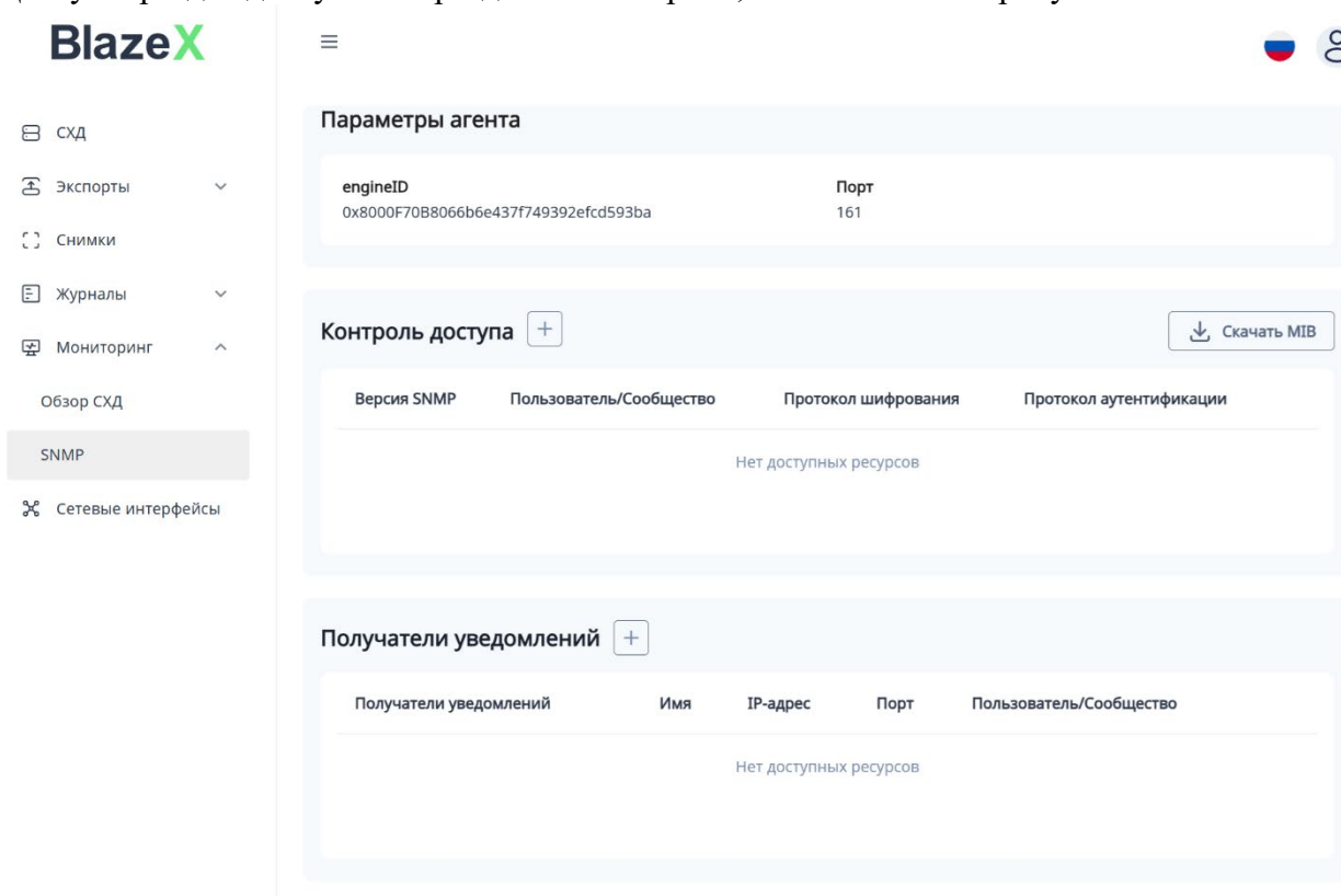
Рисунок 9.11 – Раздел SNMP
