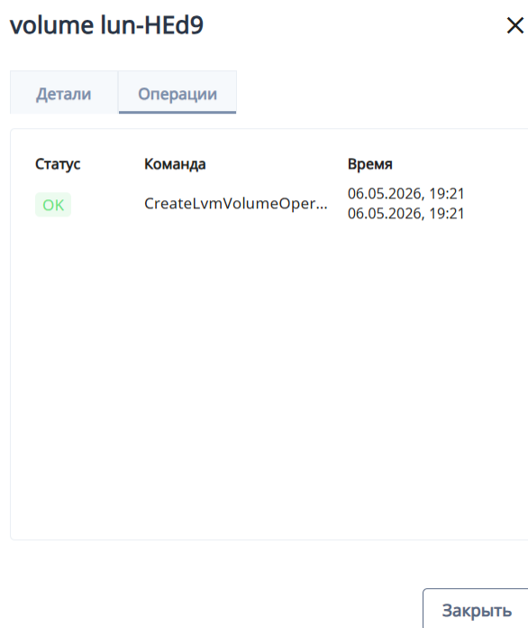
Рисунок 2.46 – Вкладка «Операции»
