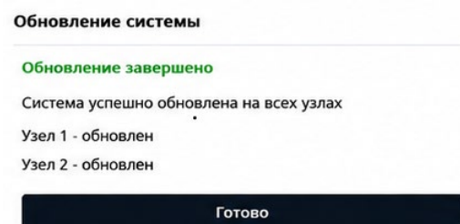
Рисунок 1.33 – Обновление завершено
