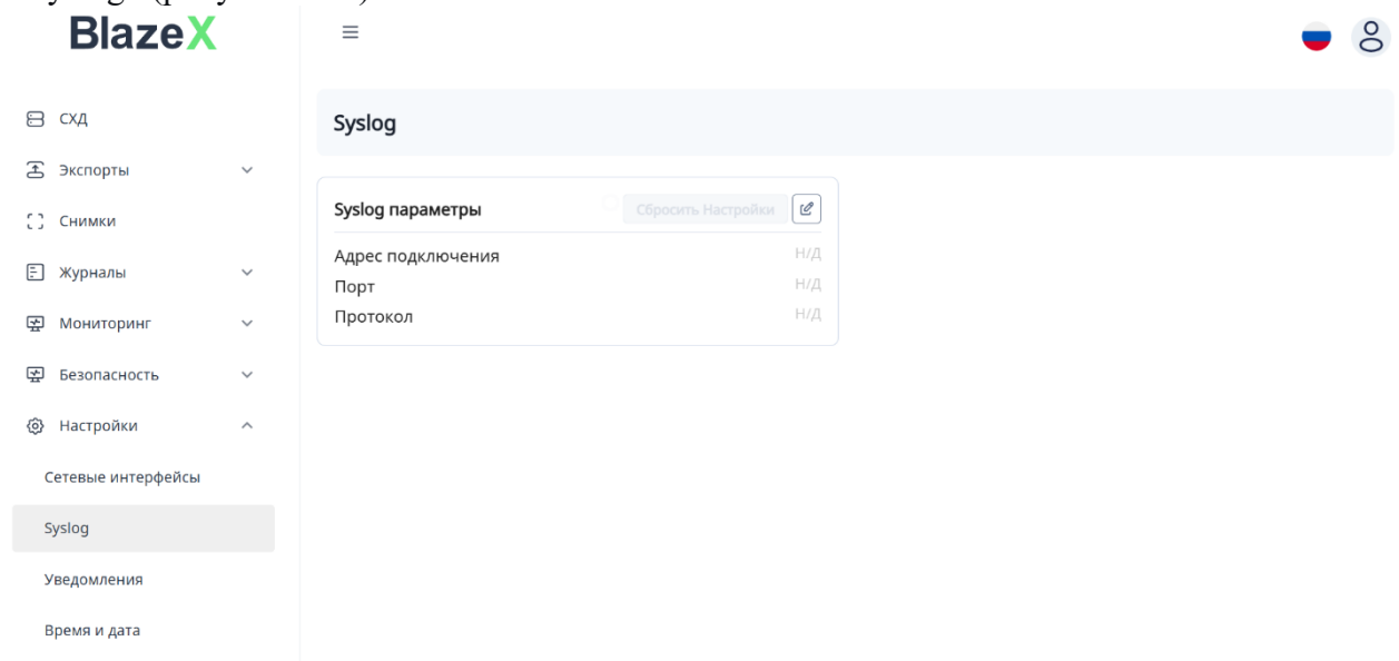
Рисунок 12.3 – Раздел «Syslog»
