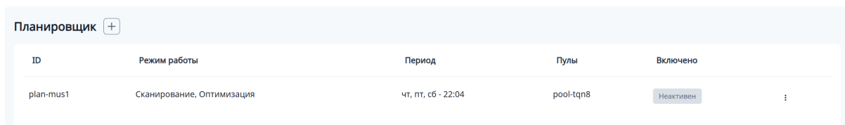
Рисунок 5.10 – Выключенное расписание
