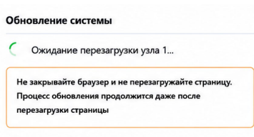
Рисунок 1.29 – Перезагрузка узла 1
