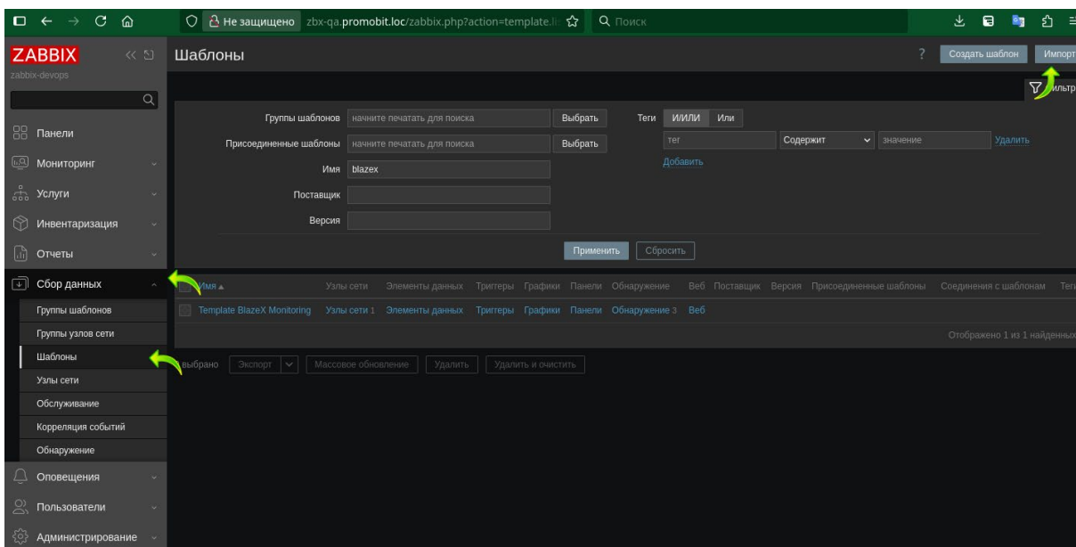
Рисунок 9.37 – Добавление шаблона
